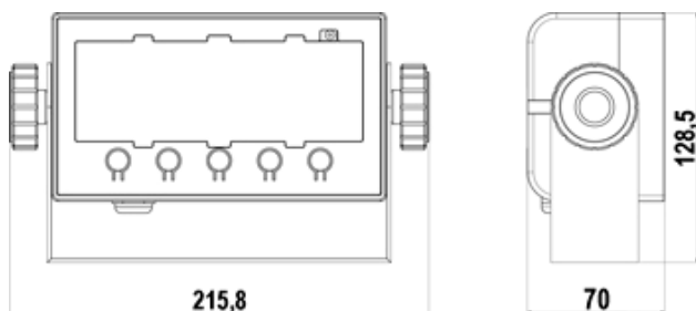
DFWL: Méretek [mm].
