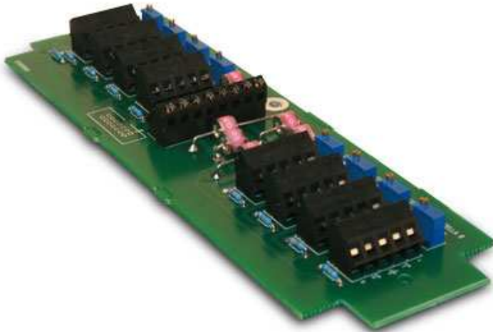
JC8QSA: kötöző és arányosító kártya 8 bemenettel.
